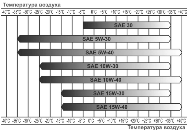
Рис. 4. Выбор масла
